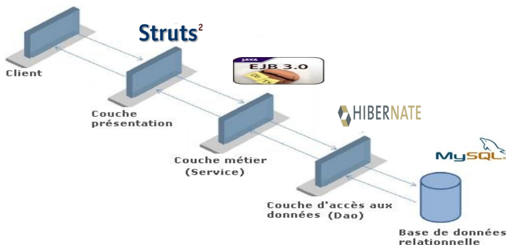
Figure 11 : Framework utilisés
